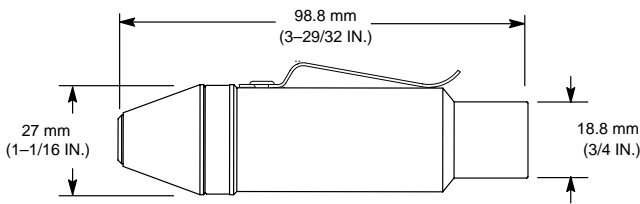
DIMENSIONS HORS TOUT • GESAMTABMESSUNGEN • DIMENSIONES GENERALES • DIMENSIONI COMPLESSIVE FIGURE 4
